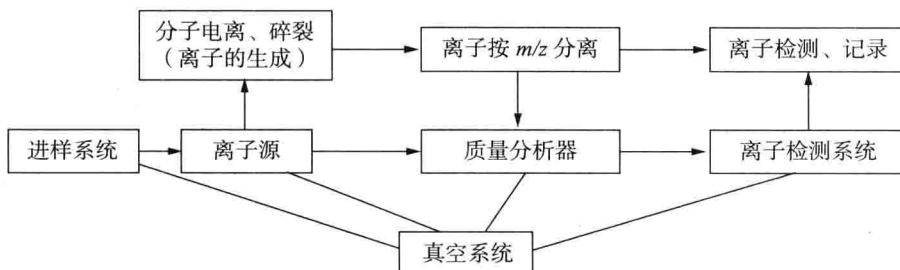
图 1.2 质谱计的构造和功能
