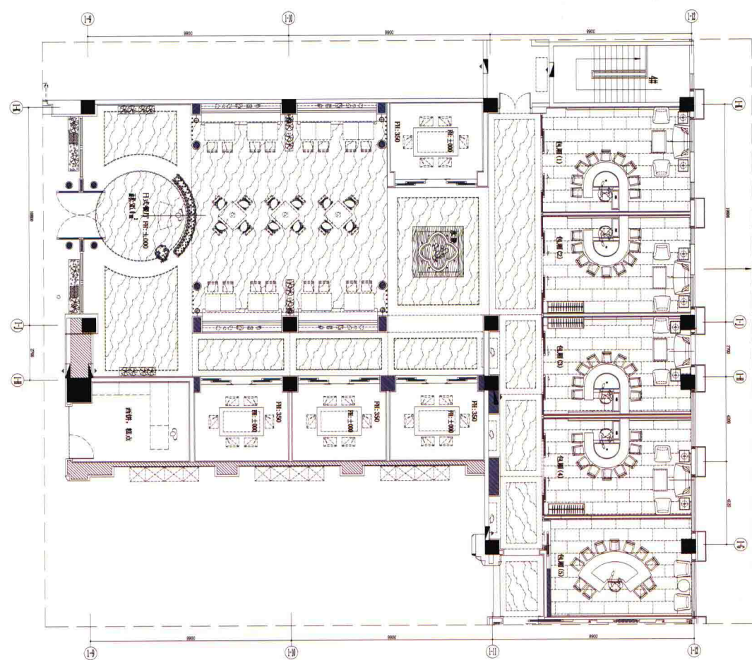
一层平面图
