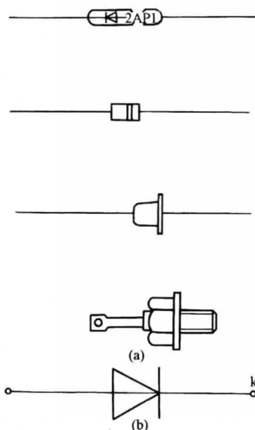
图 1-3 晶体二极管外形和符号
