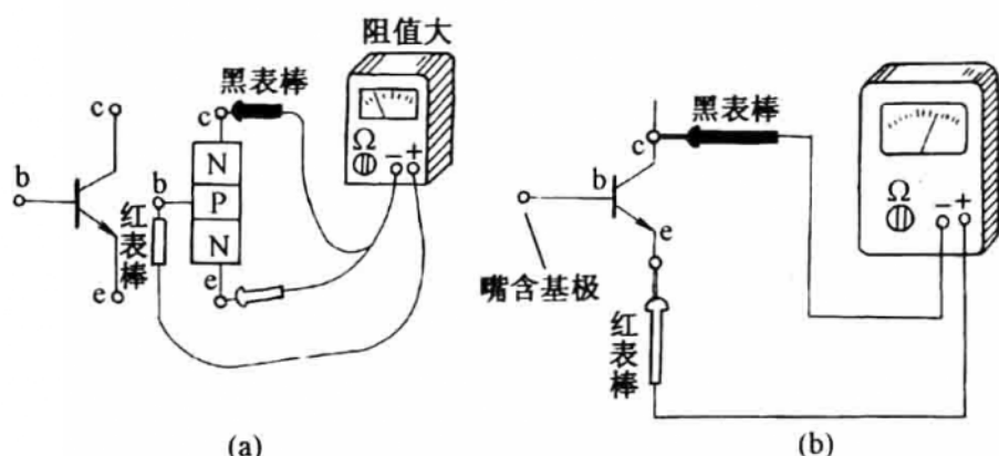
图 1-5 三极管管脚的判定 (a) 基极的判定；(b) 集电极的判定
