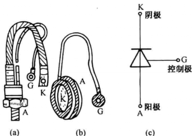
图 1-6 晶闸管的外形和符号 (a) 螺栓式；(b) 平板式；(c) 晶闸管的符号
