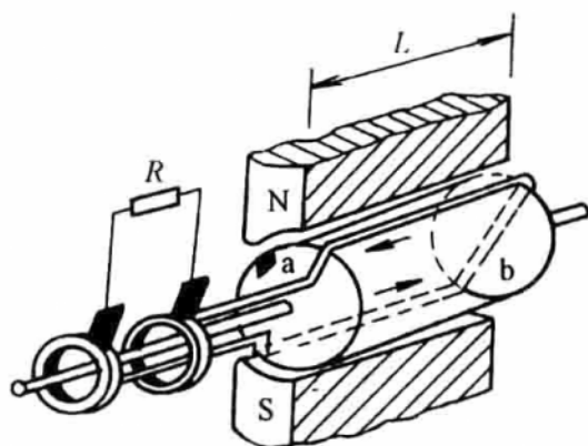
图 1-1 交流发电机结构示意图
