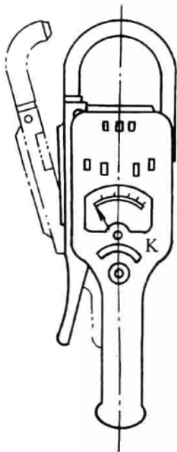
图 1-7 钳形 电流表外形
