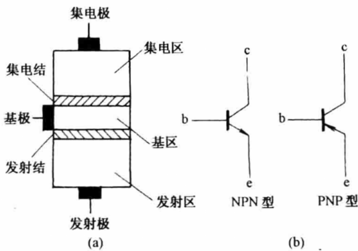
图 1-4 三极管的结构和符号 (a) 结构；(b) 符号
