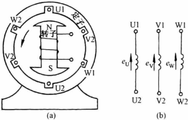
图 1-2 三相交流发电机示意
