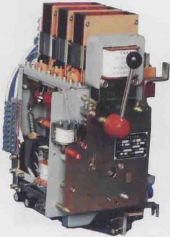
DWX15系列万能式断路器
