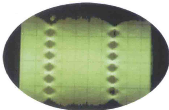
示波器上显示的6个“眼睛”
