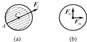
图 1.10 圆柱形铰链的约束力
