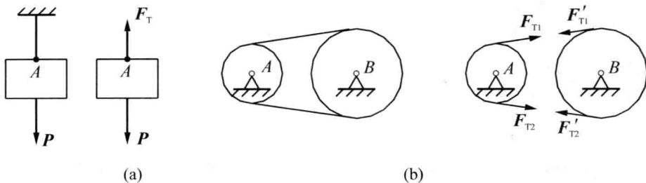
图 1.8 柔体约束
