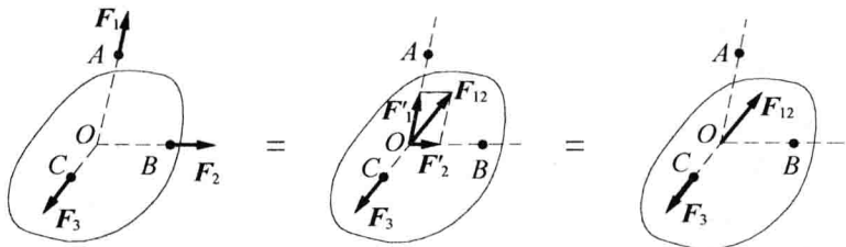
图 1.5 三力平衡汇交定理
