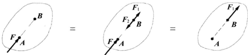
图 1.4 力的可传性
