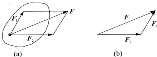
图 1.2 力的平行四边形法则和三角形法则
