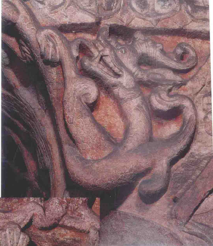
图版二二 第6窟中心塔柱南面下层东侧反顾金翅鸟
