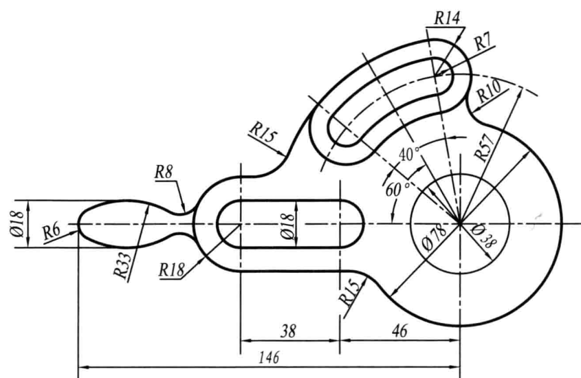
挂 轮 架
