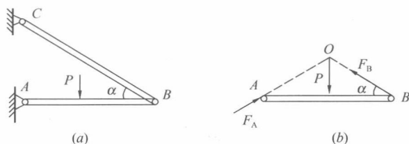
图 8-3 三力平衡必汇交
