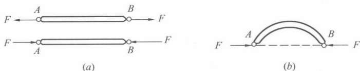
图 8-2 二力平衡必共线
