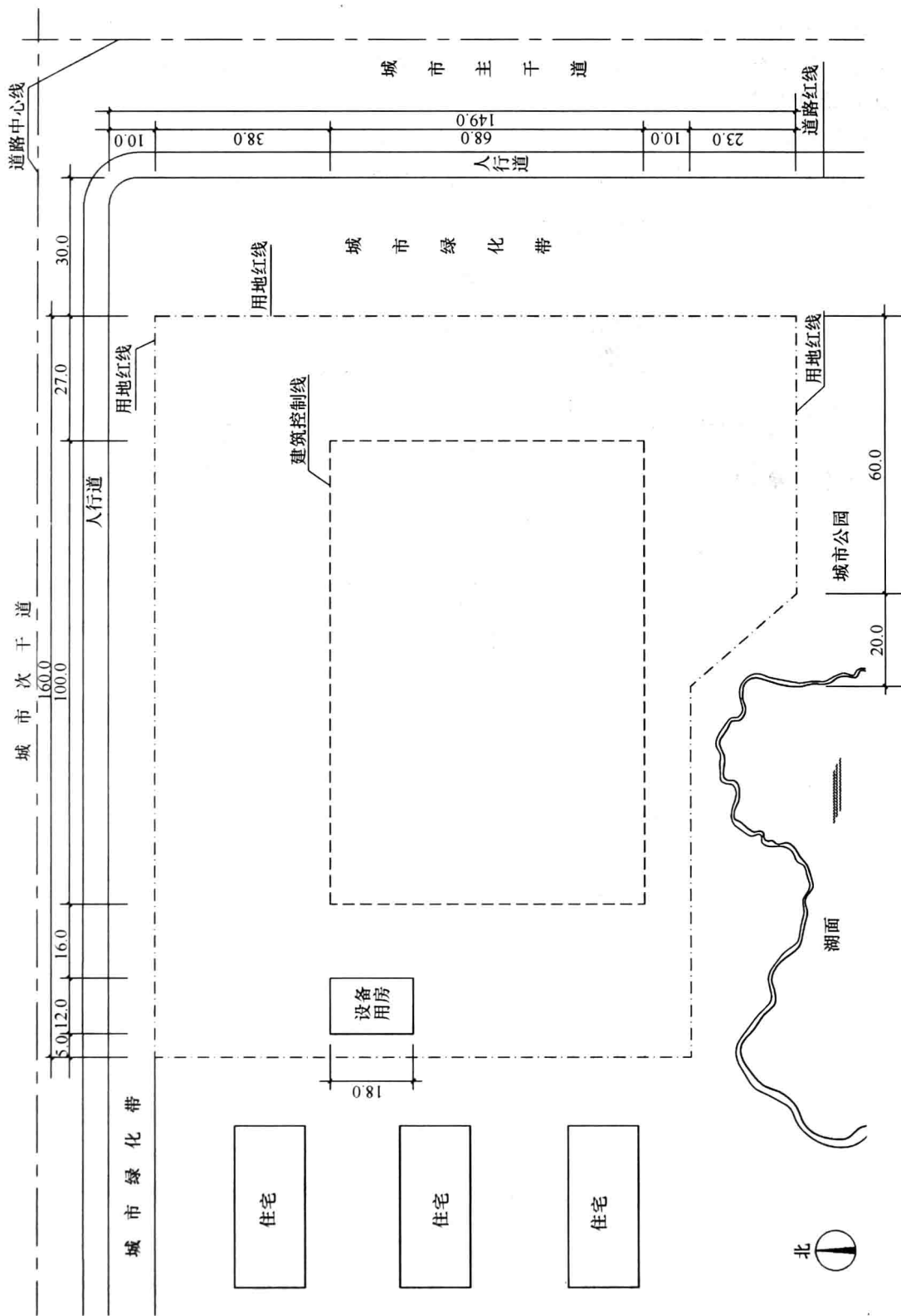
图 28-2-1 总平面图
