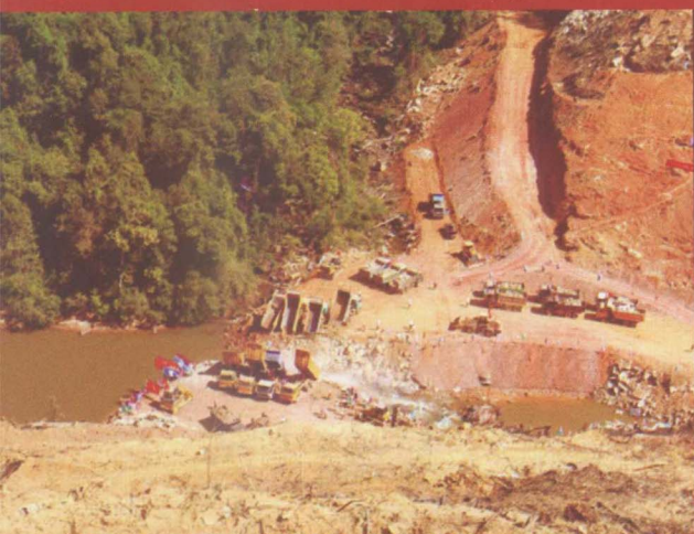
12月28日，由集团公司承建的柬埔寨额勒赛上水电站工程大江截流成功。
