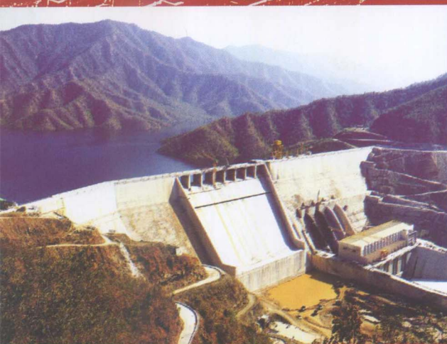
12月25日，由集团股份公司负责机电设备设计、供货与安装任务的缅甸水津水电站首台机（4号机）成功完成72小时试运行。
