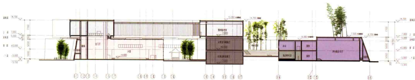
3-3 剖面图
