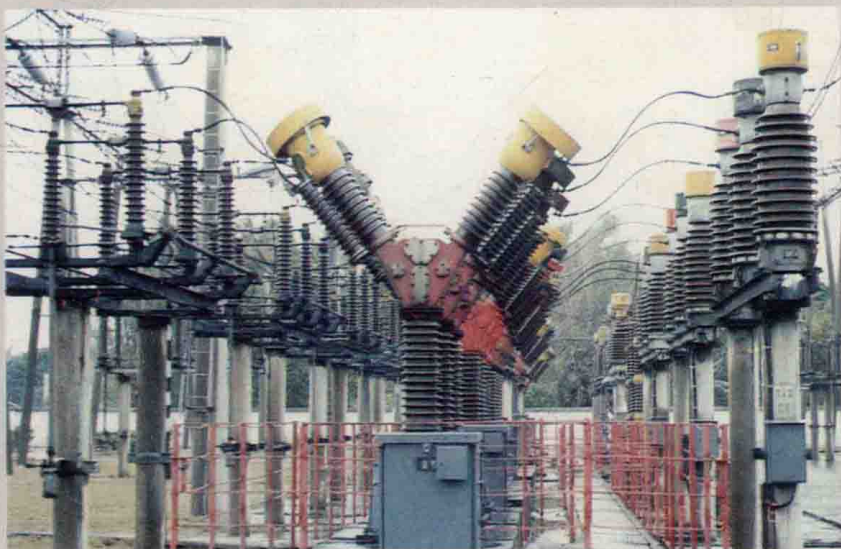
座落在鹤亭的 110 千伏设计容量 8 万千瓦的变电站
