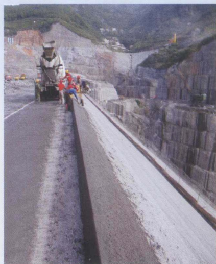
水布垭挤压边墙新工艺
