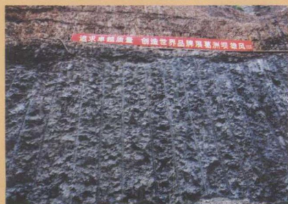
电站进水口预裂孔均匀合理
