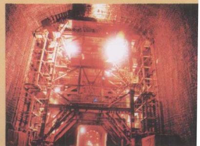
亚洲最大钢模台车屹立雄姿
