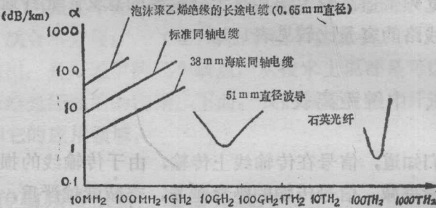
图 1.2.1 各种传输介质的损耗特性
