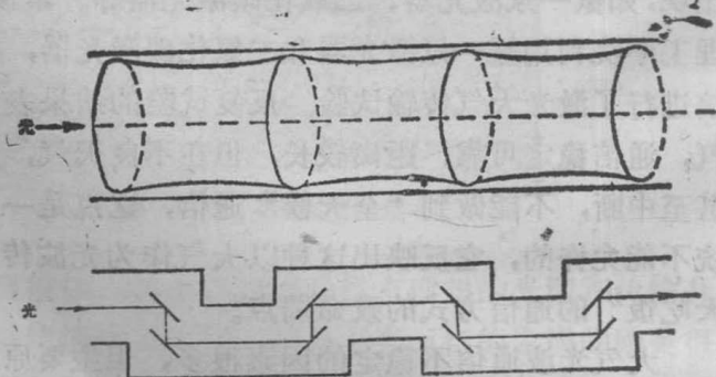
图 1.1.2 透镜波导和反射镜波导
