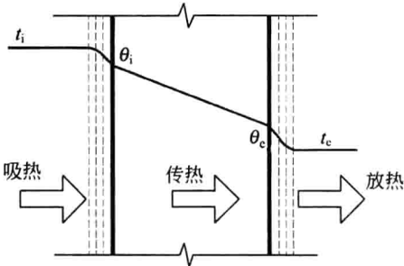
图 17-3 围护结构的传热过程
