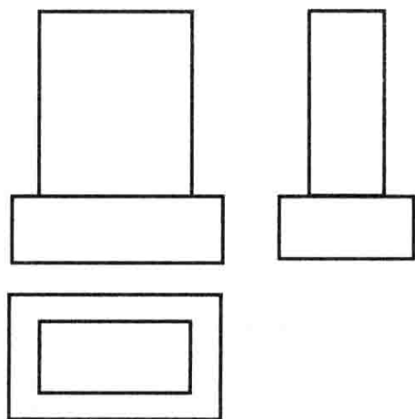
图 1-1-14 正投影图
