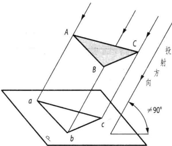
图 1-1-9 斜投影法
