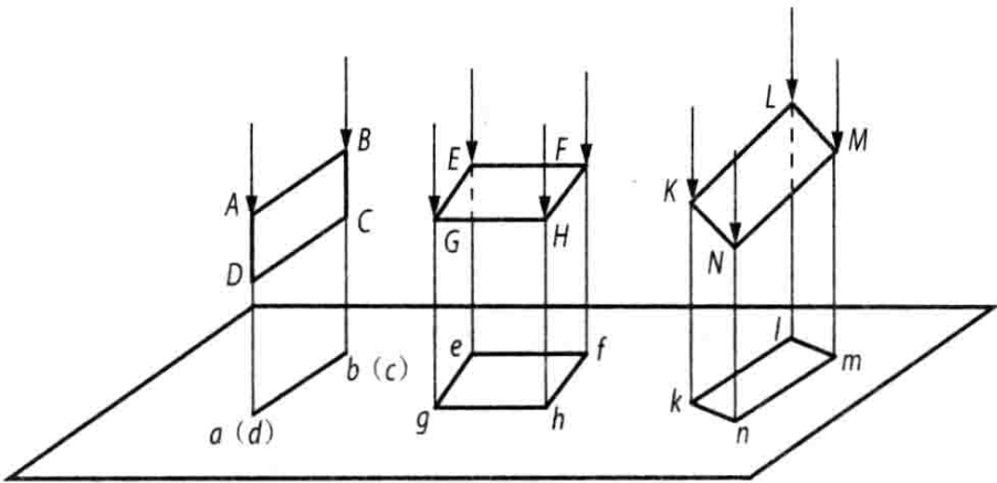
图 1-1-19 平面的正投影规律
