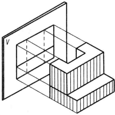
图 1-1-7 物体的投影
