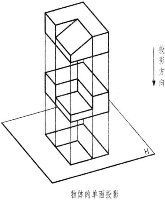
图 1-1-20 物体的单面投影图
