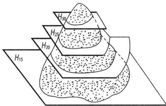
图 1-1-16 标高投影图的形成
