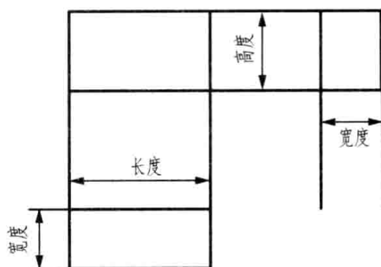
图 1-1-25 立面投影图的规律
