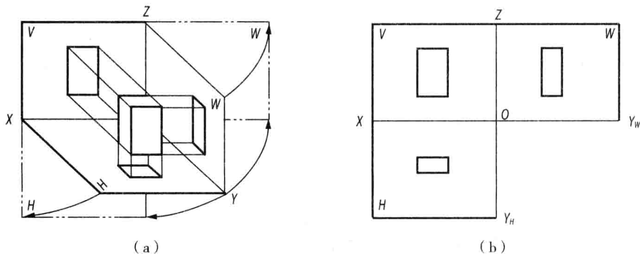
图 1-1-23 投影面的展开
