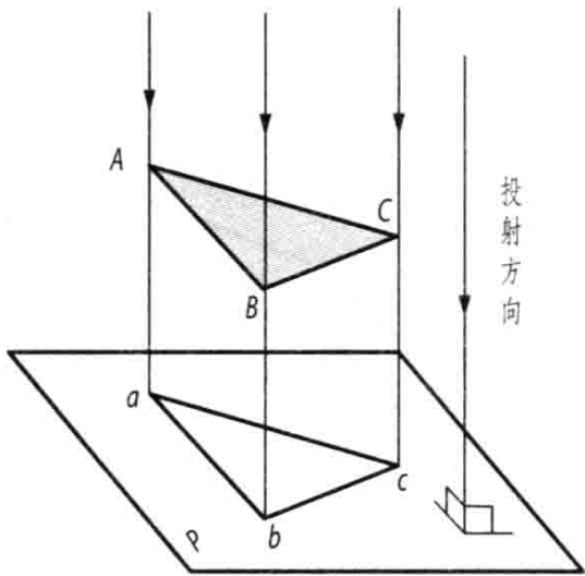
图 1-1-10 正投影法
