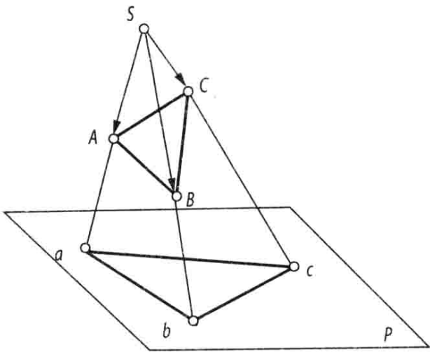
图 1-1-8 中心投影法
