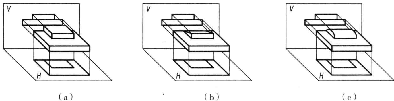
图 1-1-21 物体的双面投影图
