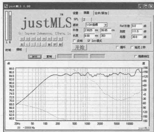
图1.8 用电脑软件连接音箱输出测试得到的曲线
