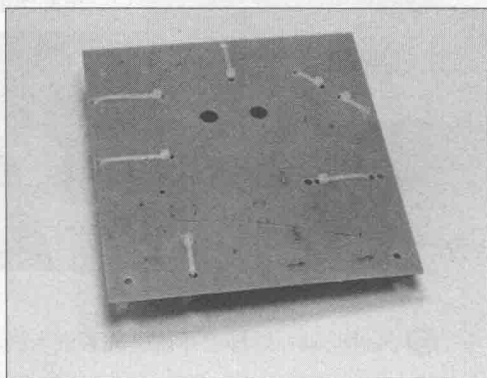
图1.6 固定大体积元件用尼龙扎带
