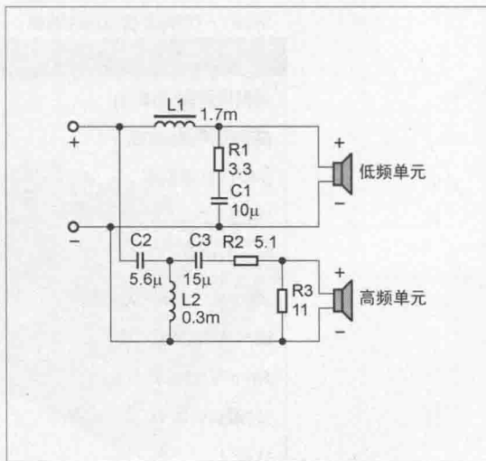
图1.3 分频器电路
