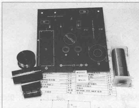
图1.5 分频器的PCB及元件
