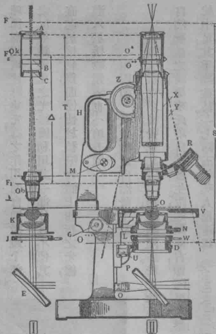
第四圖 顯微鏡中光線之進路
