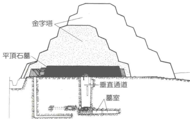
◎ 卓瑟金字塔剖面图
