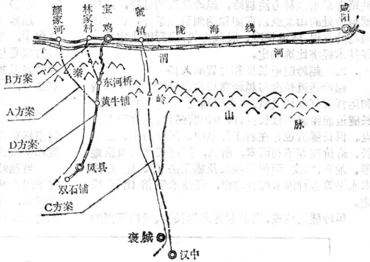
图1.1.4 宝成线秦岭垭口选择示意图
