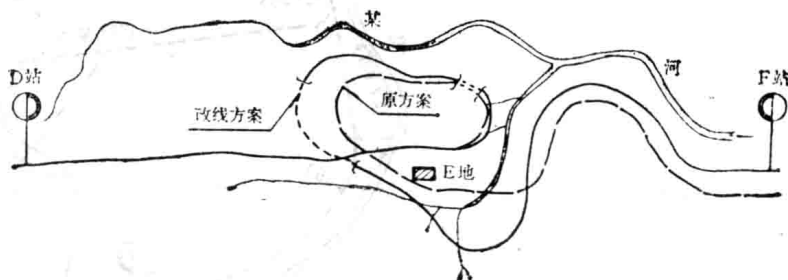
图1.1.7 河谷展线示意图
