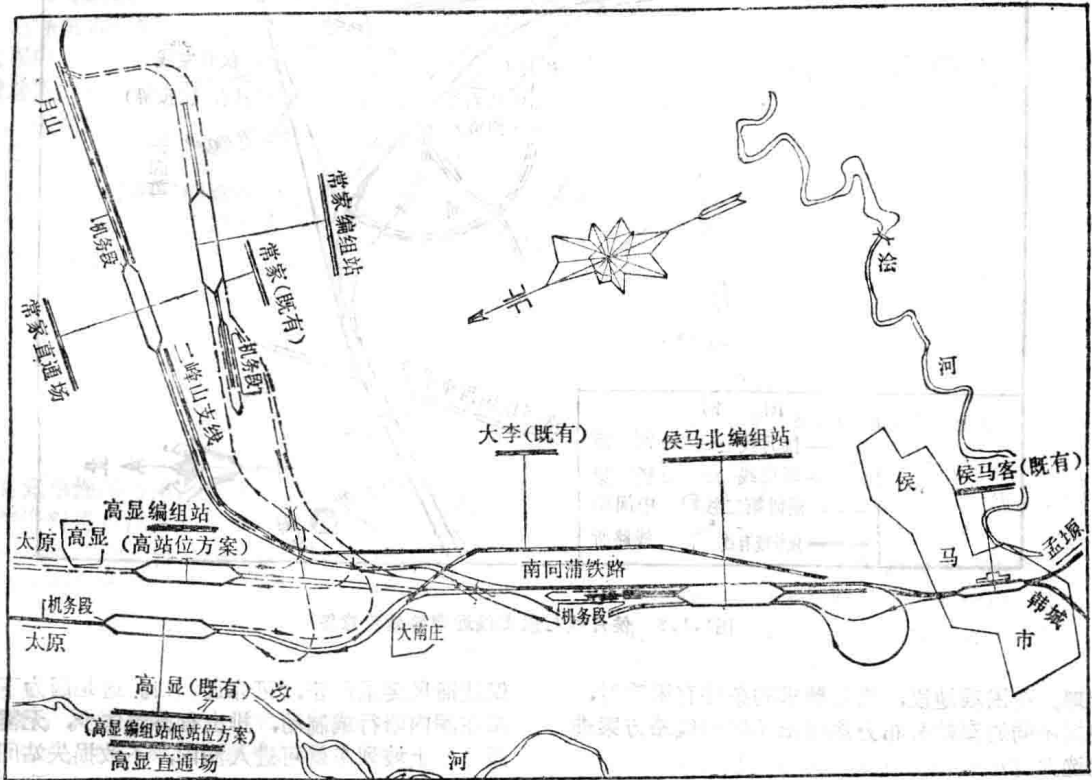
图1.1.2· 侯月线侯马北编组站接轨示意图
