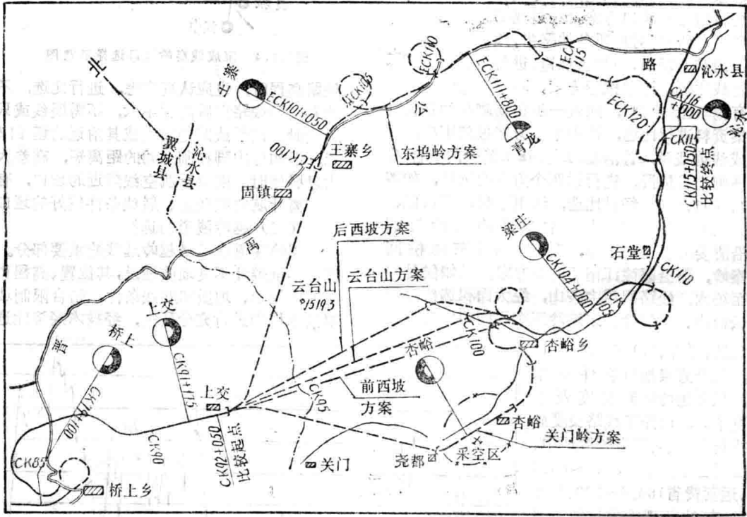
图1.1.6 侯月线中条山越岭方案比较示意图
