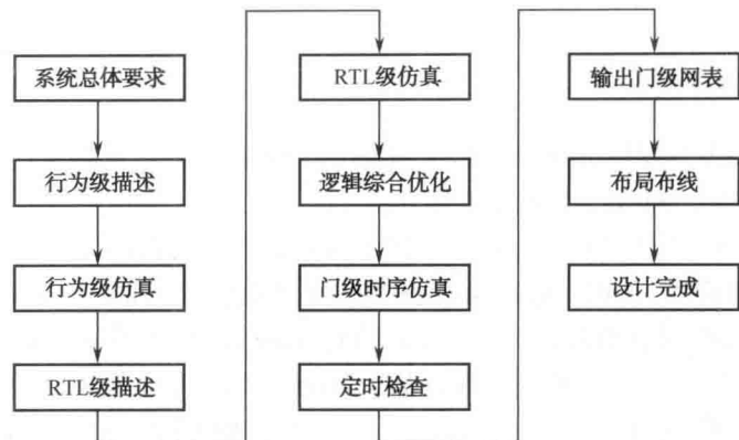
图 1-3 EDA 设计流程
