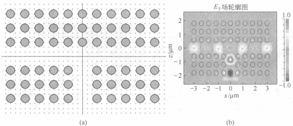
图 1.5 光子晶体波导结构和稳态光场分布示意图
