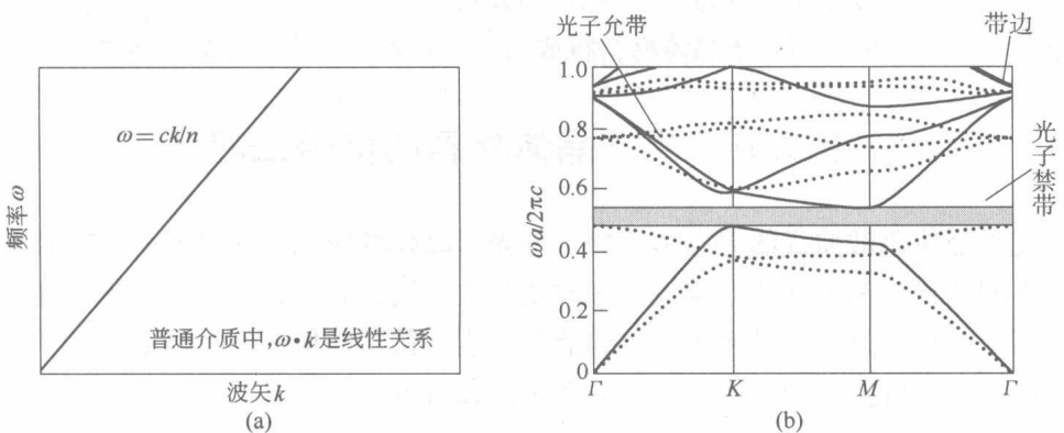
图 1.2 普通介质和二维三角晶格光子晶体的色散曲线 (a) 普通介质的色散曲线；(b) 光子晶体的色散曲线
