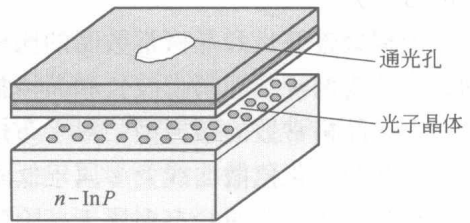
图 1.3 光子晶体激光器
