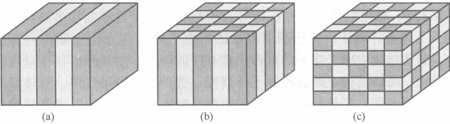
图 1.1 光子晶体结构示意图
