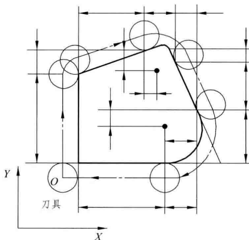
图 1-3 两坐标轮廓控制加工
