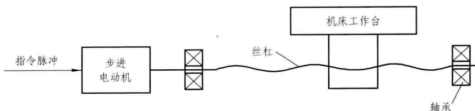
图 1-4 开环控制系统
