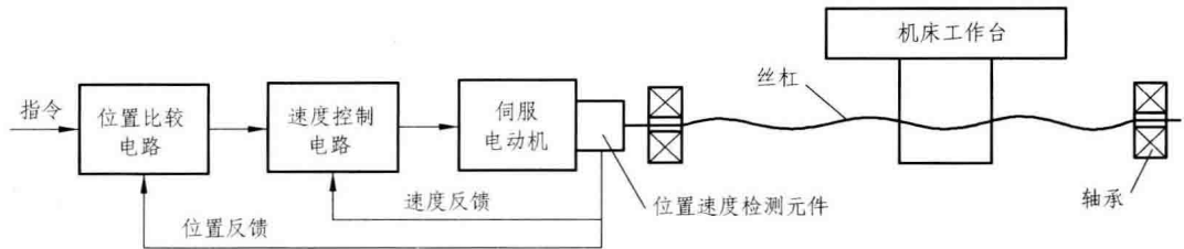
图 1-6 半闭环伺服系统
