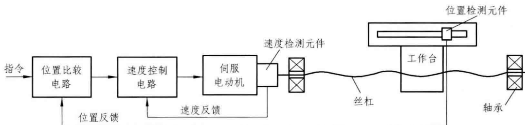
图 1-5 闭环控制系统
