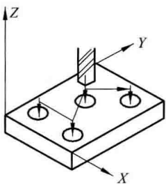
图 1-1 点位控制数控加工
