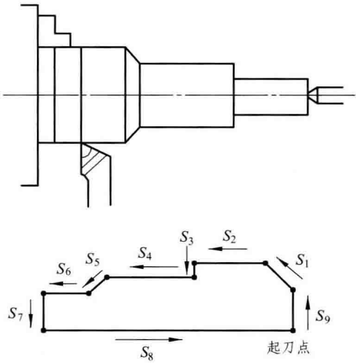
图 1-2 直线控制数控加工
