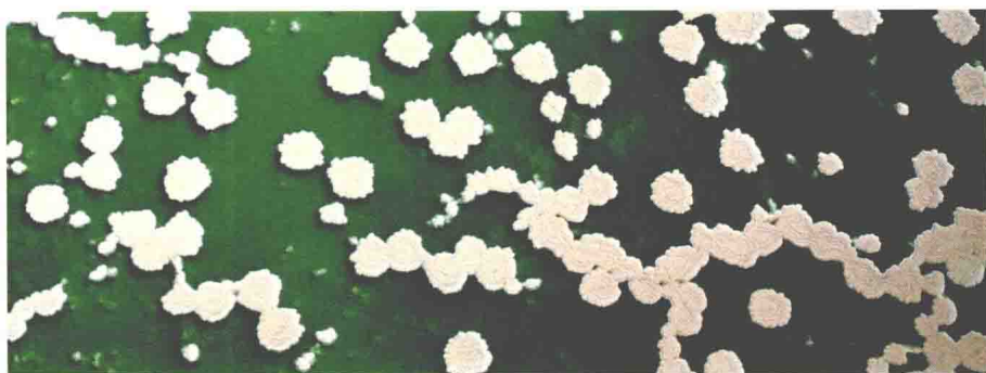
盐湖里带着的盐晶体。盐湖的主要成分是芒硝，其次是石盐。芒硝寒冷，当水温在 18\sim 20^{\circ}\text{C} 时，石盐和芒硝在水中都是不饱和的。当水温降到 5.5^{\circ}\text{C} 以下时，石盐仍然不饱和，但是芒硝会从水中析出，成为固态晶体。
