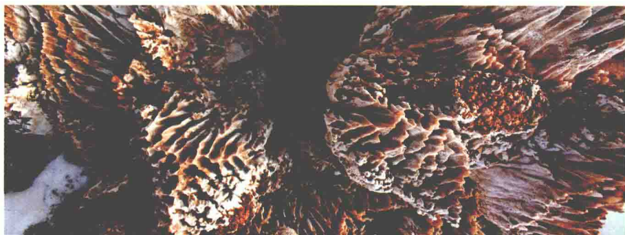
矿盐的盐苗。在温宿古盐湖遗迹中，我们看到了这样的盐喀斯特景观。因为混有泥沙等杂质，盐晶体呈现出棕红色，在常年雨水的冲刷溶解下，盐山的山体逐渐呈现出一种嶙峋峥嵘之意，看起来像一支支盐笋，也叫盐苗。
