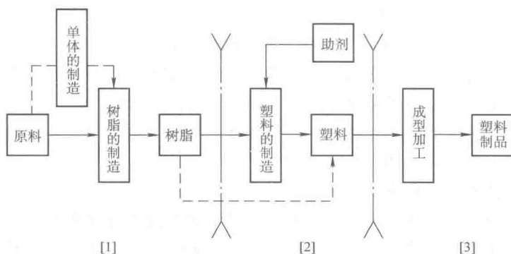
图 1-1 从原料到塑料制品的生产过程
