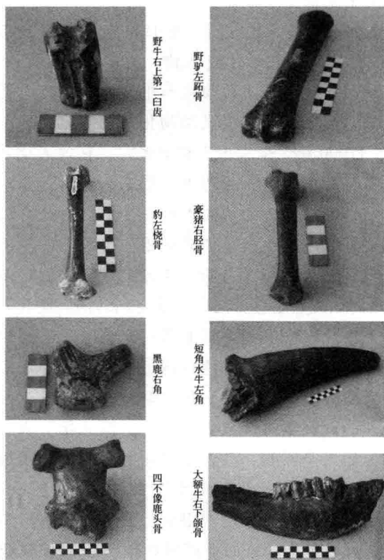
图2 泉州石狮渔民在台湾海峡捞获的哺乳动物化石
