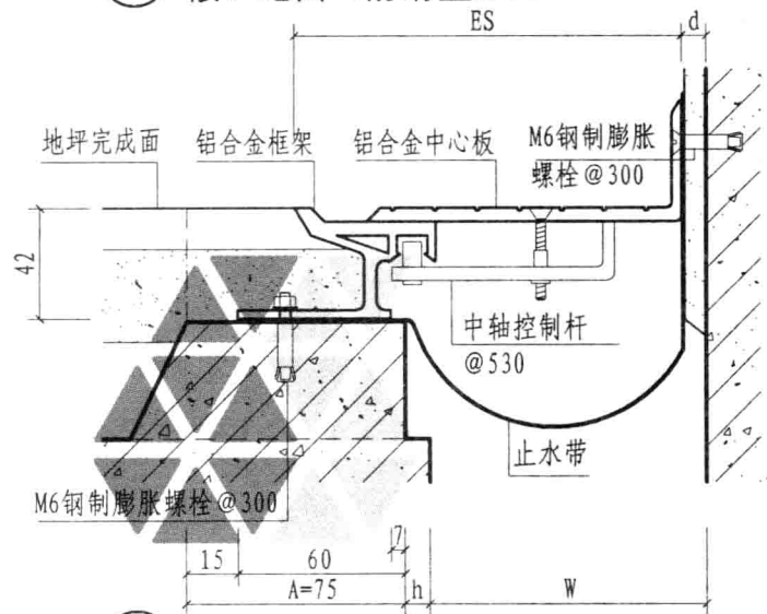
② b 楼、地面与墙面 (防滑型DJF)
