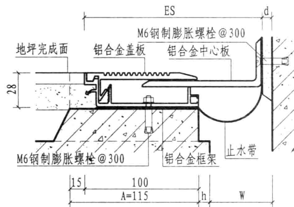
② 楼、地面与墙面（卡锁式DJK）
