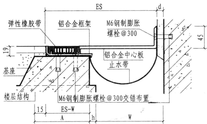
② b 楼、地面与墙面（嵌平式DJR）
