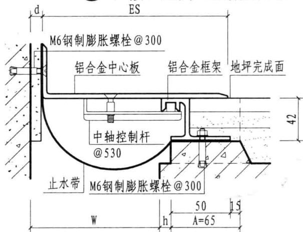
②b 楼、地面与墙面（盖板型DJL）
