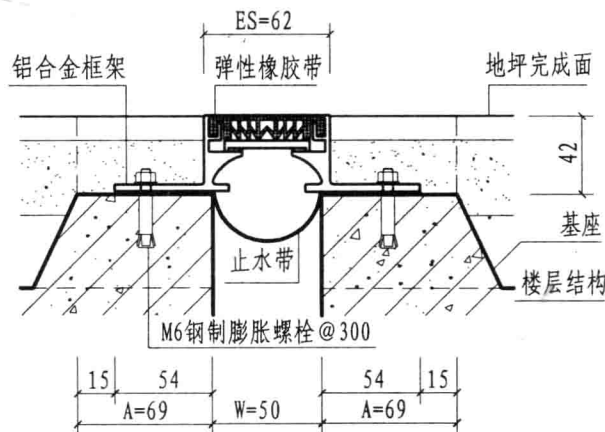
② 楼、地面（嵌平式DPR-50）
