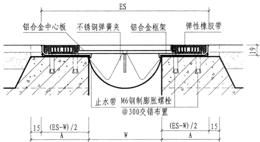
① 楼、地面（双列嵌平式DPRSC）
