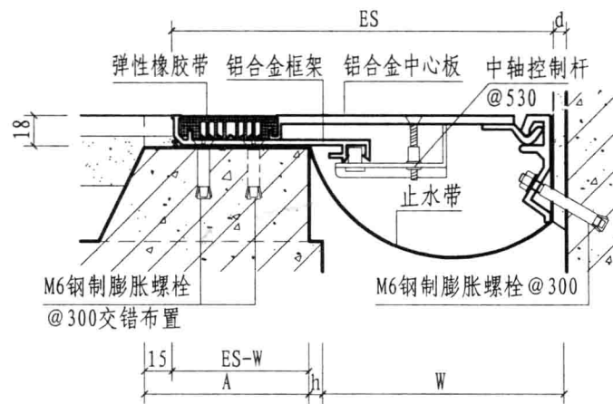
③ 楼、地面与墙面（嵌平式DJC）
