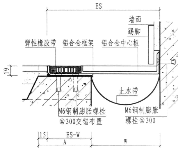
② a 楼、地面与墙面（嵌平式DJRSC）
