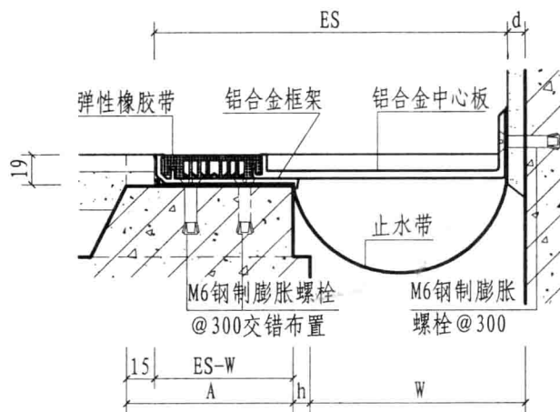
② b 楼、地面与墙面（嵌平式DJRSC）
