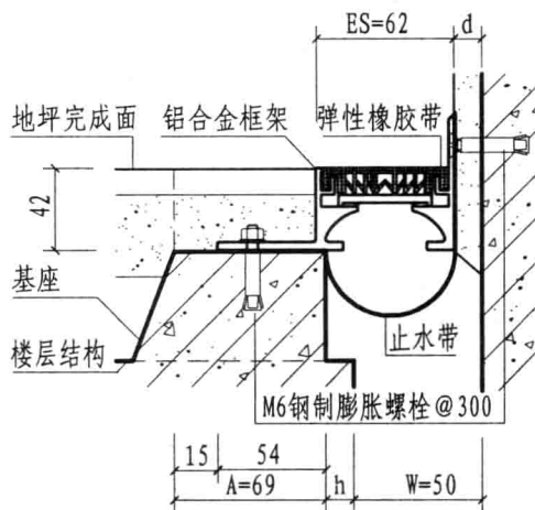
④ 楼、地面与墙面（嵌平式DJR-50）
