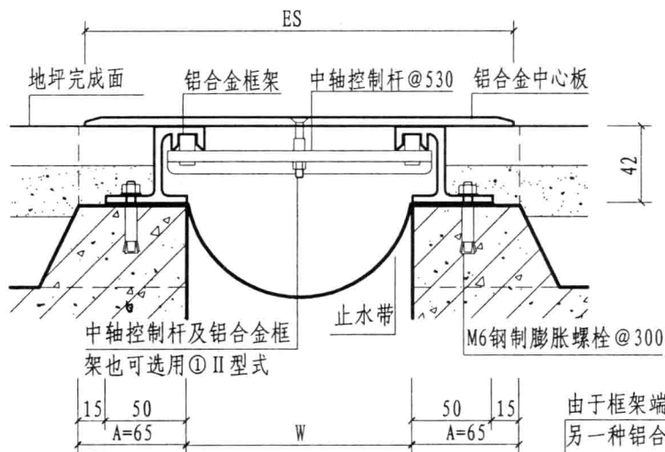
①a 楼、地面（盖板型DPL）
