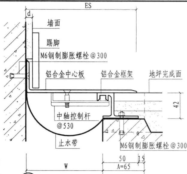
②a 楼、地面与墙面（盖板型DJL）
