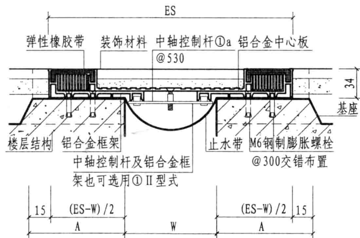
① a 楼、地面（嵌平式DPRS）
