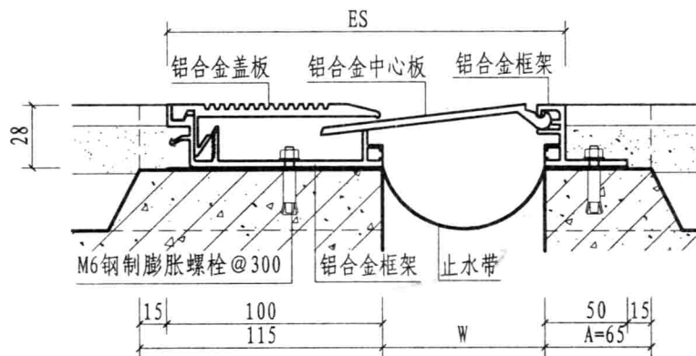
③ 楼、地面（卡锁式DPC）
