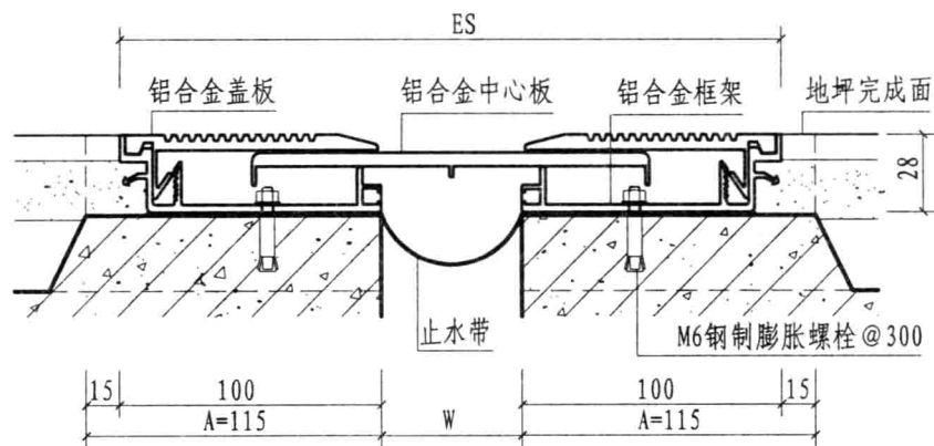
① 楼、地面（卡锁式DPK）
