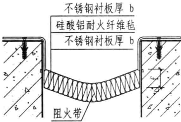
阻火带安装示意图
