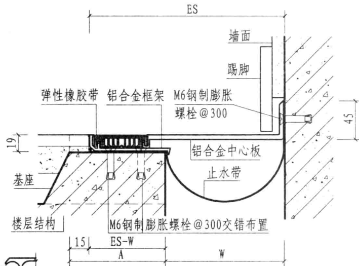
② a 楼、地面与墙面（嵌平式DJR）
