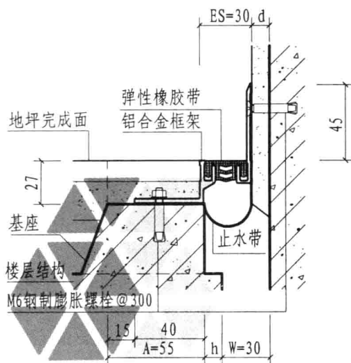
③ 楼、地面与墙面（嵌平式DJR-30）
