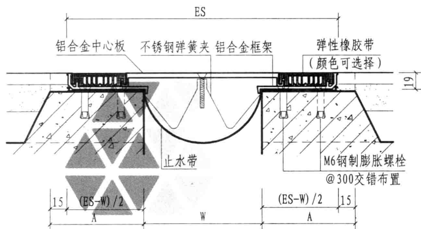
② 楼、地面（嵌平式DPRC）
