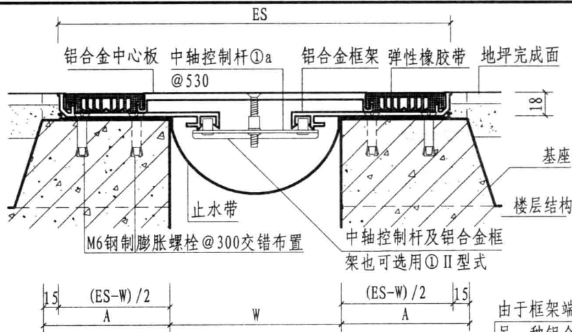
① a 楼、地面（嵌平式DPR）
