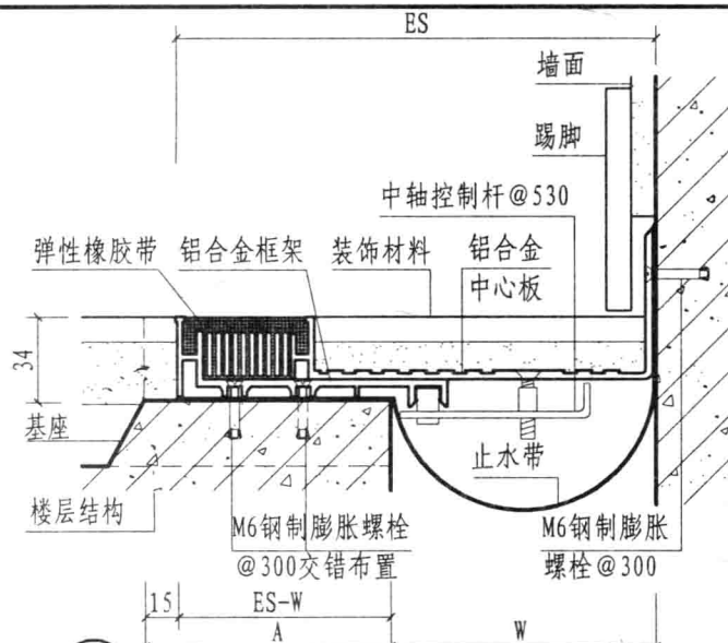
② a 楼、地面与墙面（嵌平式DJRS）
