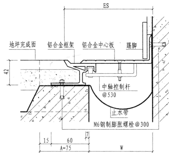
② a 楼、地面与墙面 (防滑型DJF)
