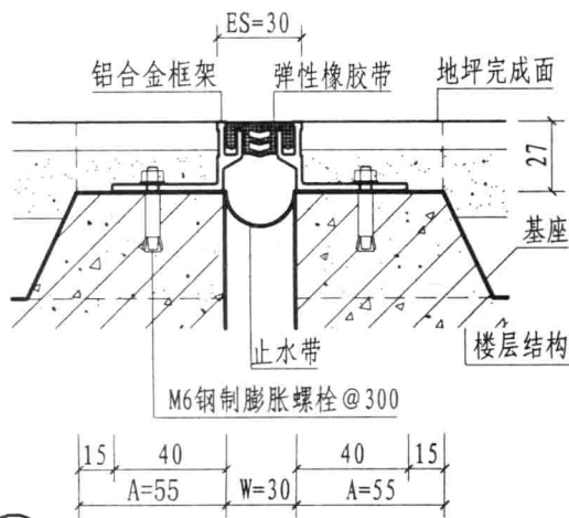
① 楼、地面（嵌平式DPR-30）
