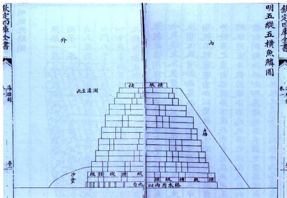
明代五纵五横鱼鳞石塘图 (《海塘录》)
