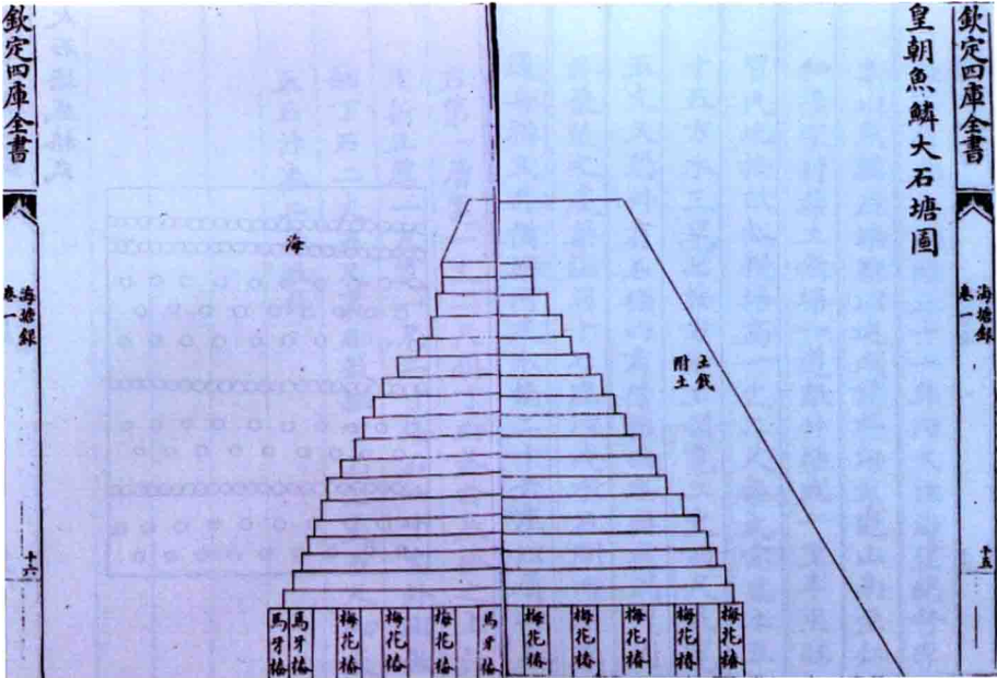
清代魚鱗大石塘圖 《海塘錄》
