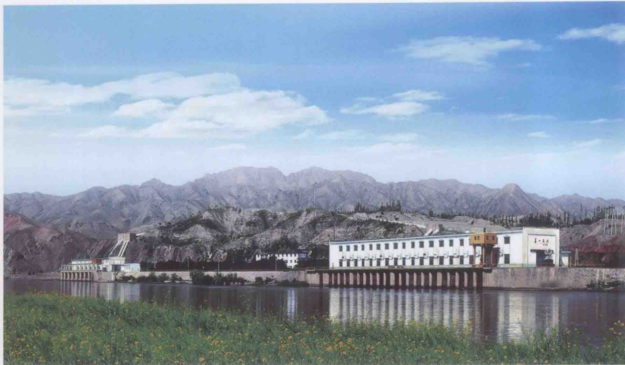
图 7 甘肃省景电工程一泵站
