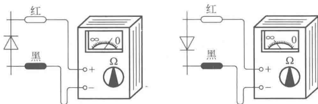
图 1-5 用指针式万用表测试二极管
