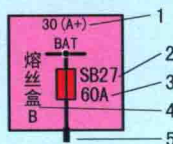
熔丝符号
