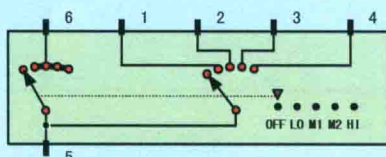
鼓风机调速开关
