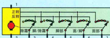
鼓风机调速开关
