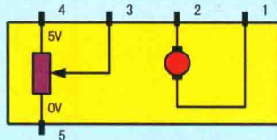
风板电动机
