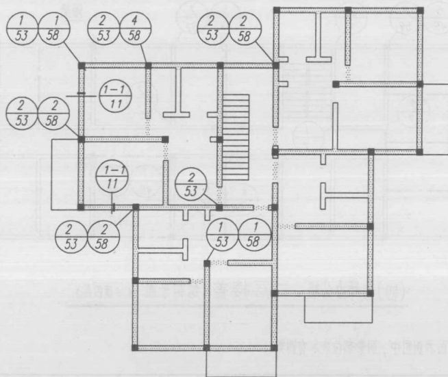
(二) 点式住宅 屋盖 结构平面 (7度六层)
