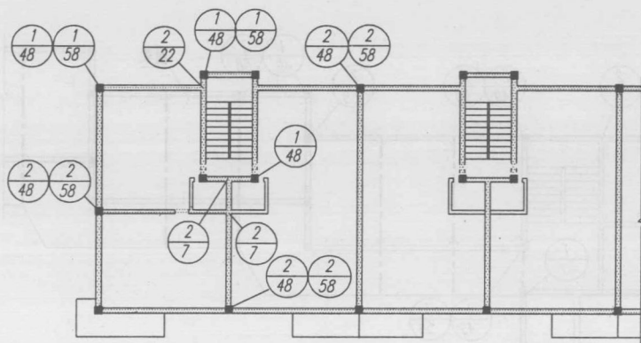
(一) 大开间住宅 楼盖 结构平面 (7度五层)
