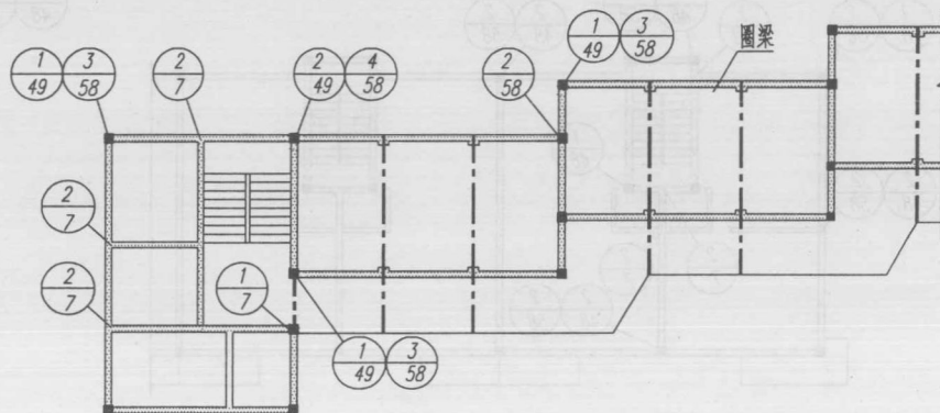
(三) 挑廊教学楼 屋盖 结构平面 (6度四层)
