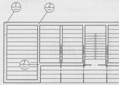
节点选用示例 (6度三层楼房的楼盖)
