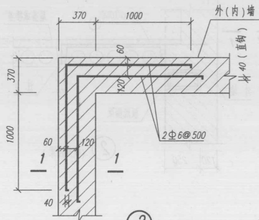
② (370 墙转角)
