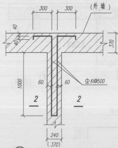
④ (370 外墙)
