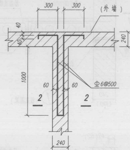
③ (240 丁字墙)
