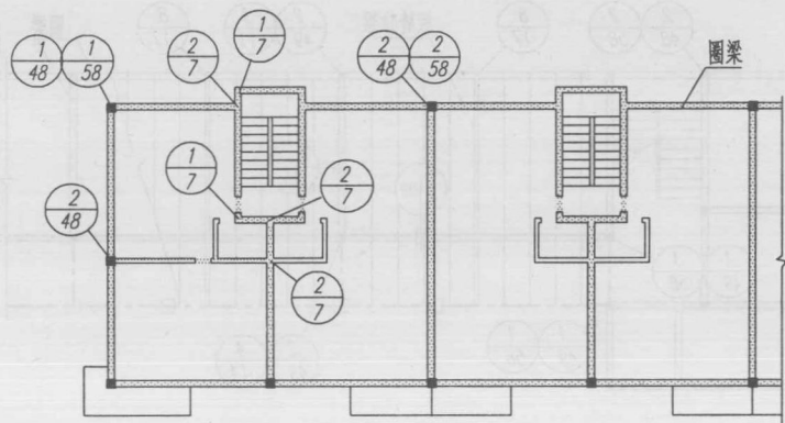
(一) 大开间住宅 屋盖 结构平面 (6度五层)
