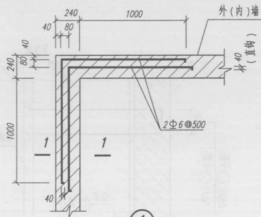
① (240 墙转角)
