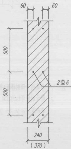
2 — 2
