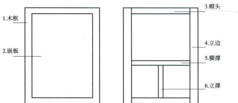
图 1-2-12 木框结构
