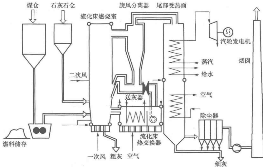
图 1-2 循环流化床锅炉系统示意
