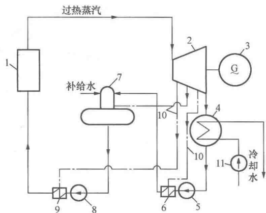
图 1-1 火力发电厂生产过程示意
