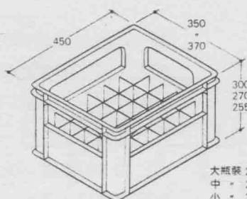
啤酒瓶搬運箱
