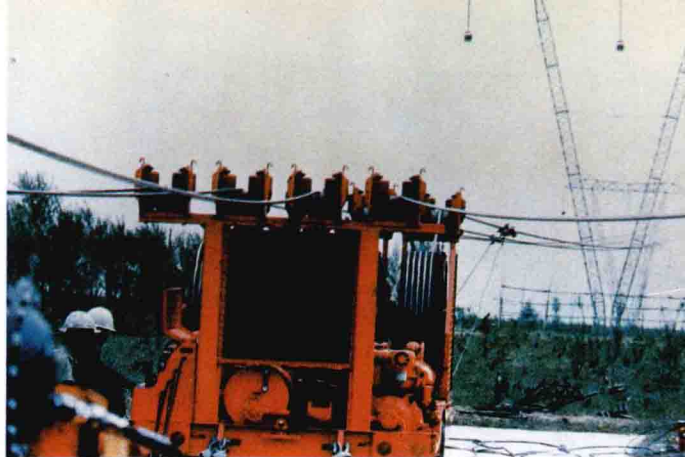
省送变电公司使用进口张力放线进行 500 千伏线路施工放线
