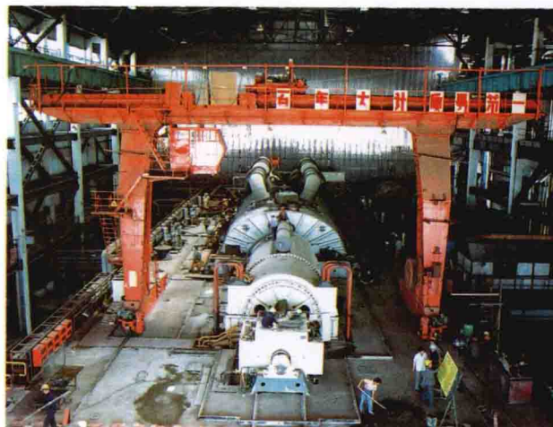
电建工人安装捷制 50 万千瓦机组
