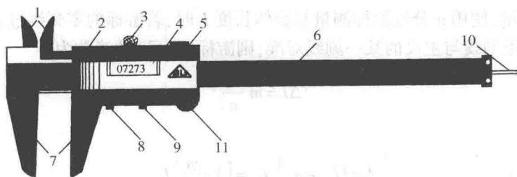
图 1-4 数字显示卡尺
