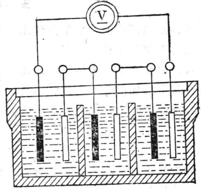
图4—1—2 用测量电压法检查内壁破裂
