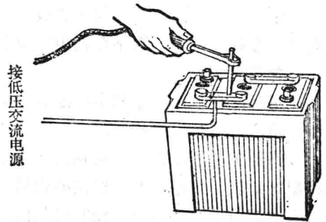
图 4—1—7 用低压交流电源焊接连条
