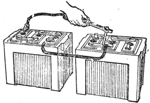
图 4—1—6 用炭棒电极焊接连条
