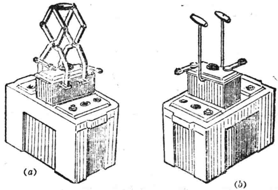
图4—1—5 拆极板组的专用工具
