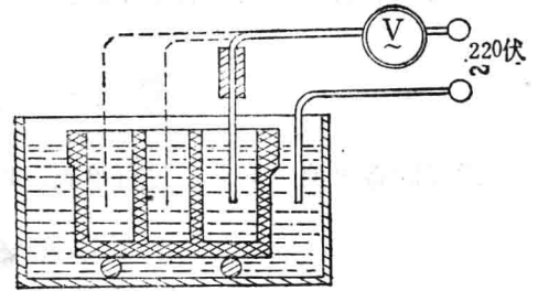
图4—1—3 用交流电检查蓄电池壳
