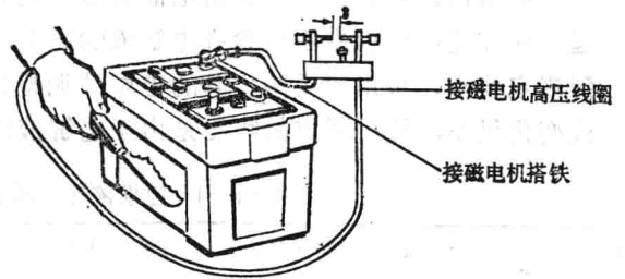
图4—1—1 用高压电检查蓄电池壳体裂纹
