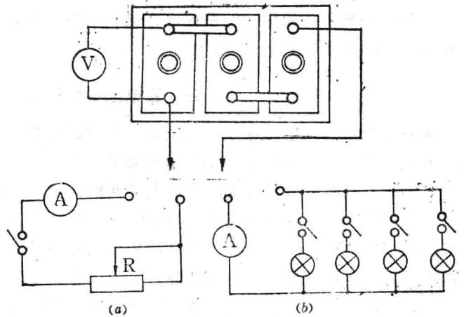
图4—1—4 蓄电池的放电方法
