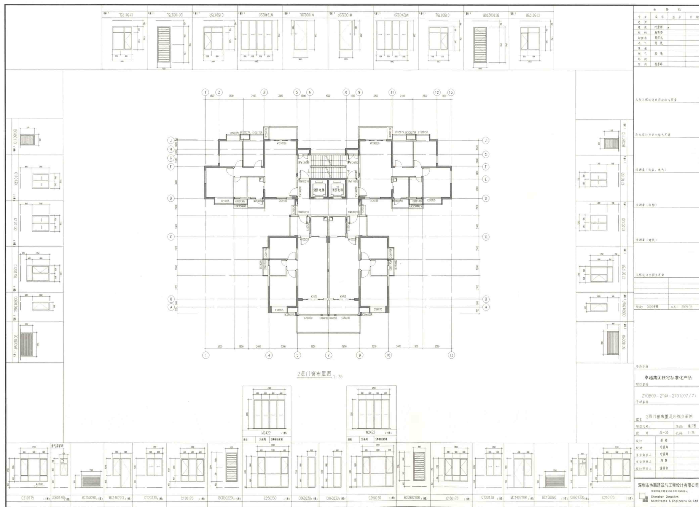
门窗布置及外视立面图
