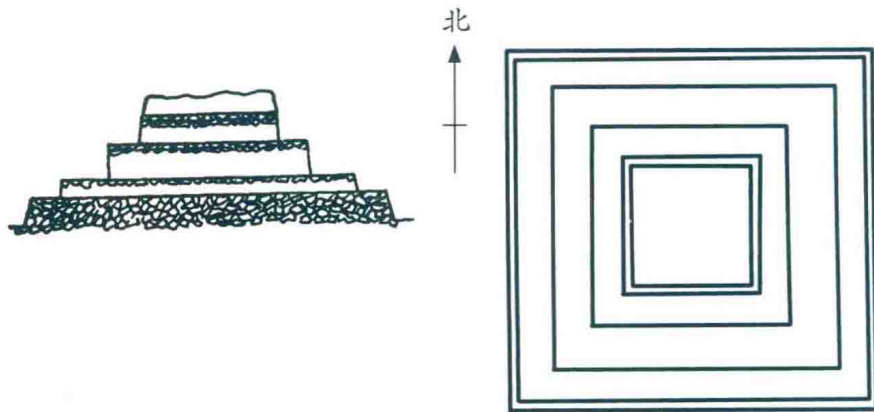
图3 塔形封土平面、侧视图
