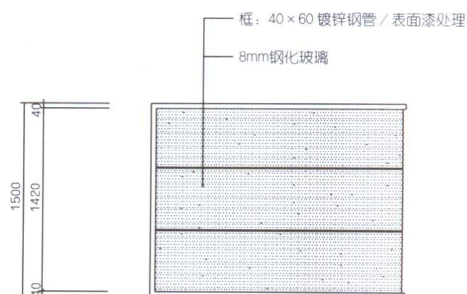
前视图
