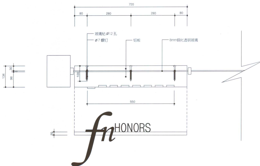
立面图
