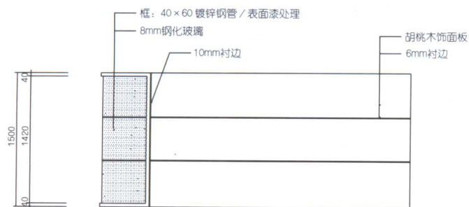
侧视图
