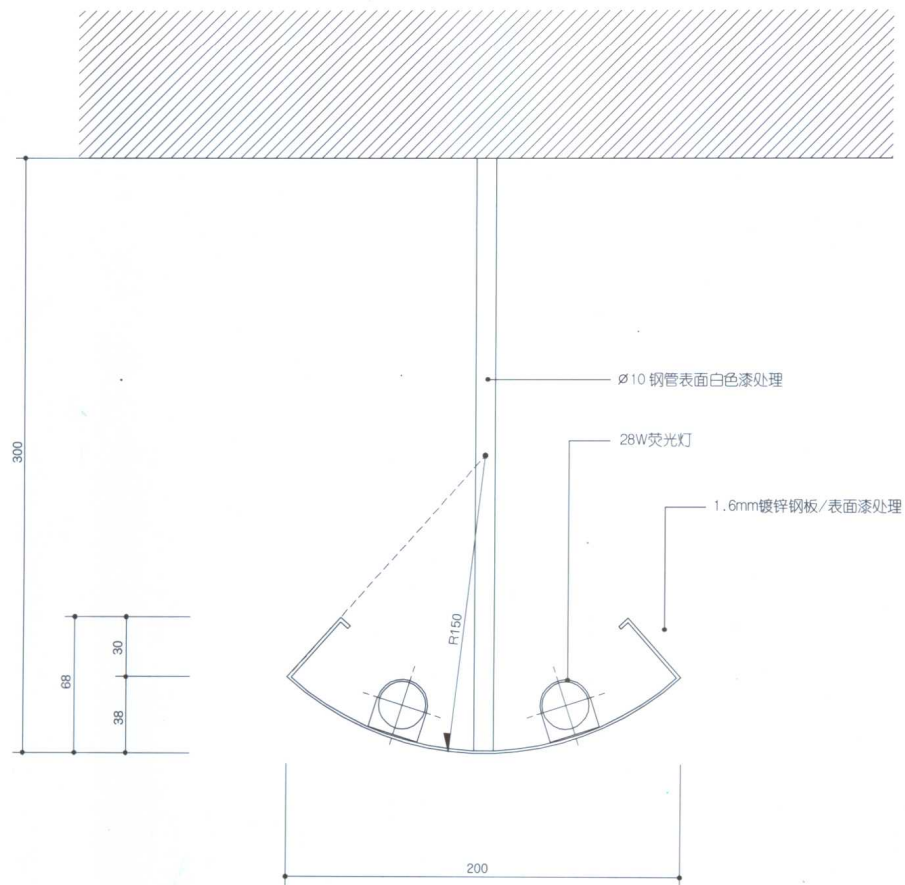
吊灯-剖面图
