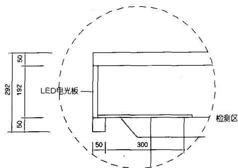
详图 A
