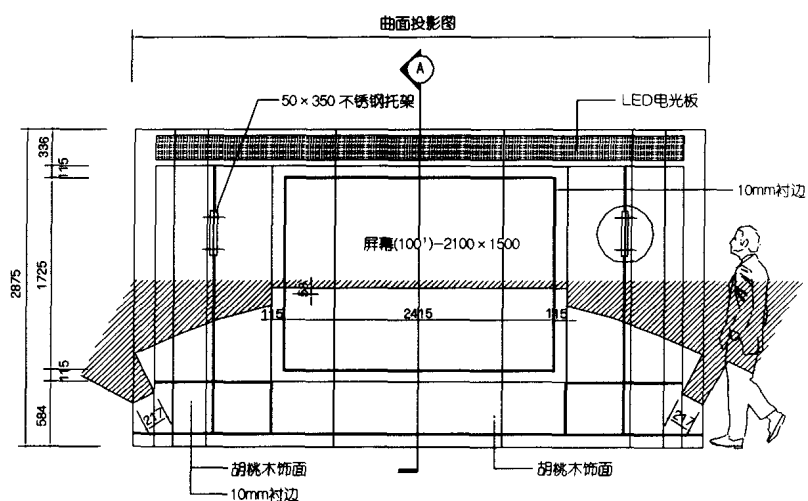
立面图
