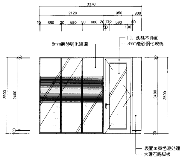
立面图
