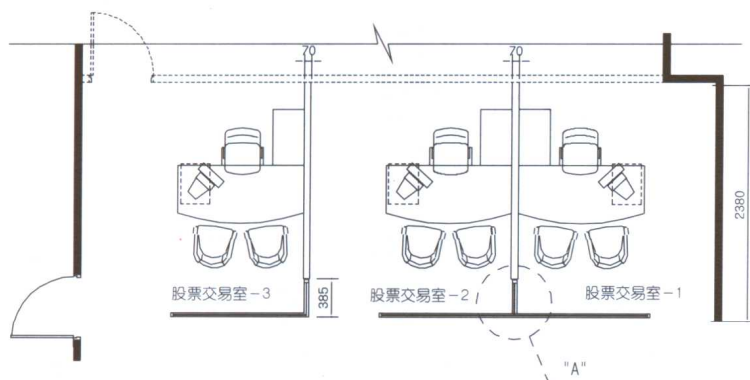
隔断平面图
