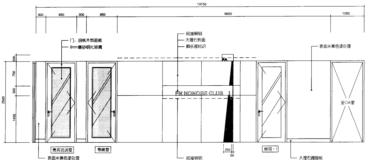
立面图
