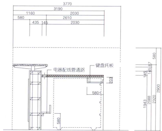
剖面图
