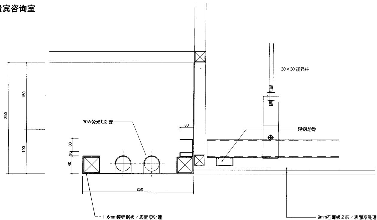
剖面图 1
