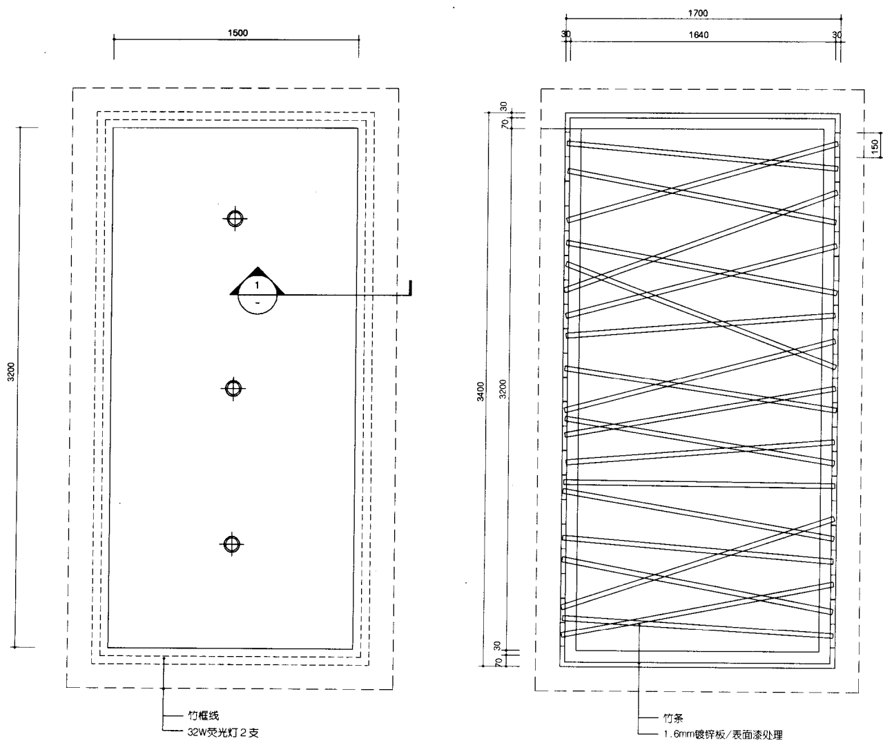
天花平面图
