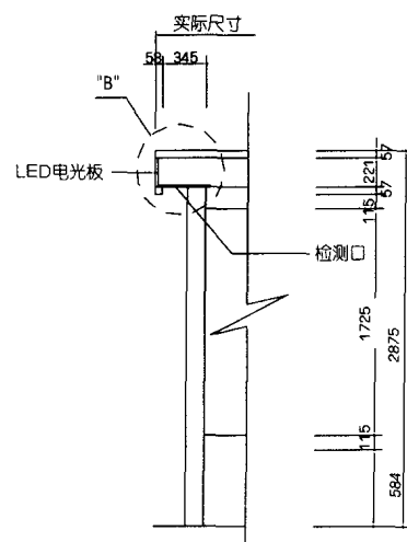
剖面图 A
