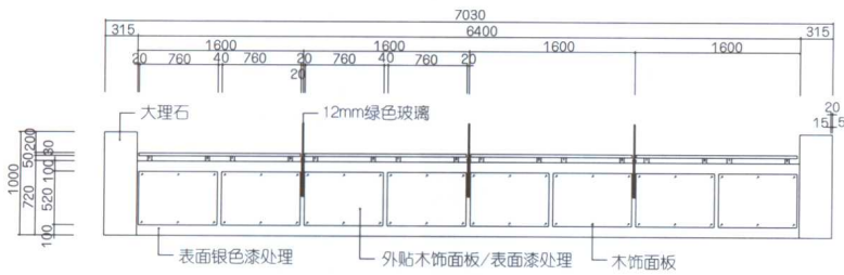
前视图
