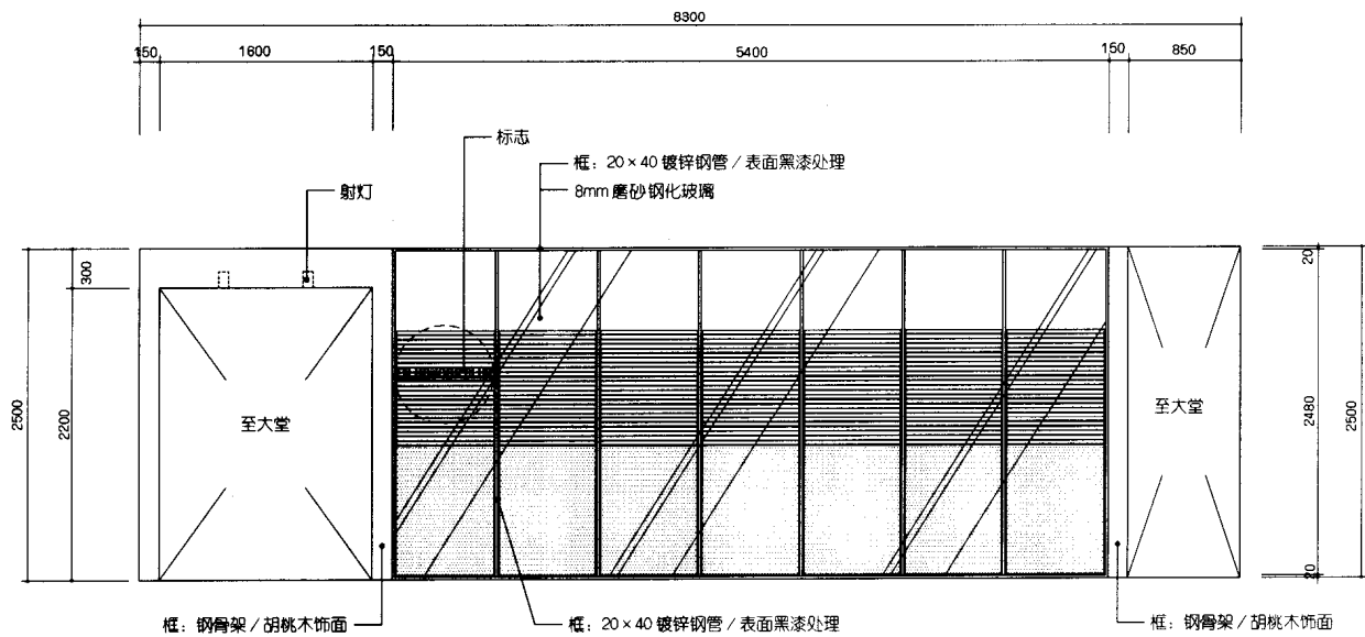
立面图
