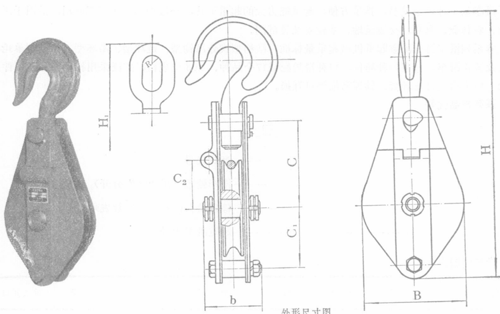
外形尺寸图
