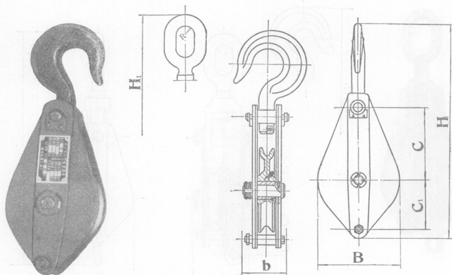
外形尺寸图
