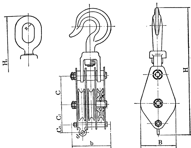
外形尺寸图
