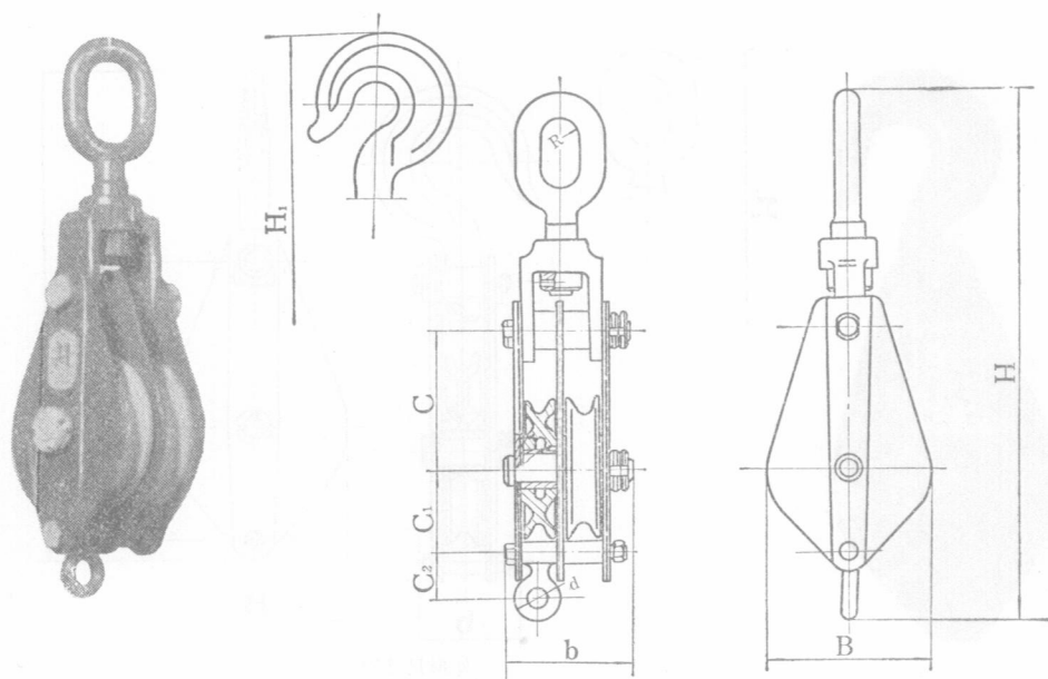
外形尺寸图
