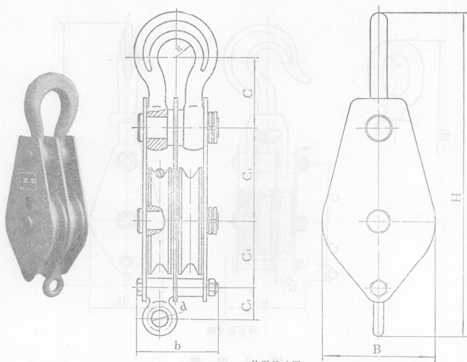
外形尺寸图
