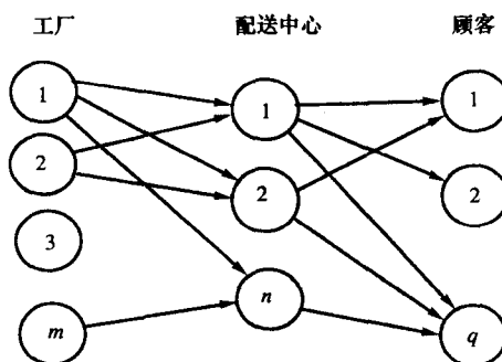
(b) 若干个配送中心的选择
