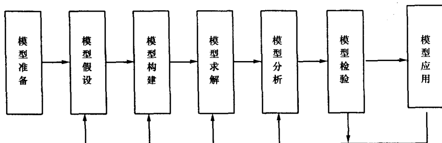
图 2-1 数学建模步骤流程图
