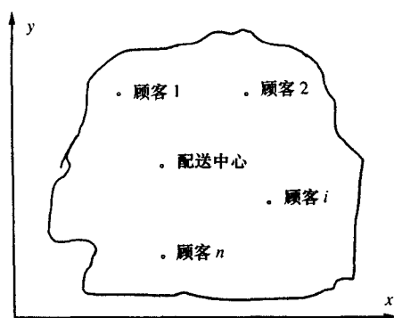
(a) 单一配送中心选址
