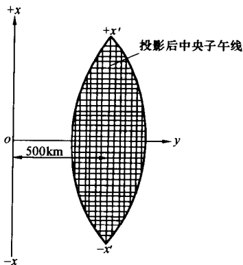
图 1-7 坐标纵轴西移
