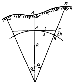
图 1-11 水平面代替大地水准面对水平距离和高程的影响
