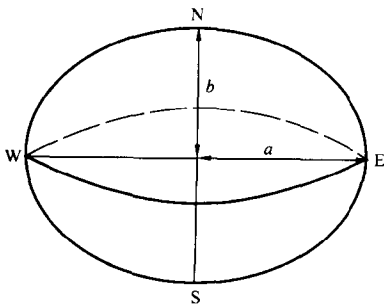
图 1-1 旋转椭球面
