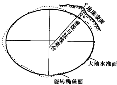
图 1-2 大地水准面和旋转椭球面
