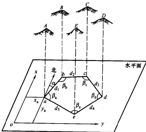
图 1-8 水平面投影
