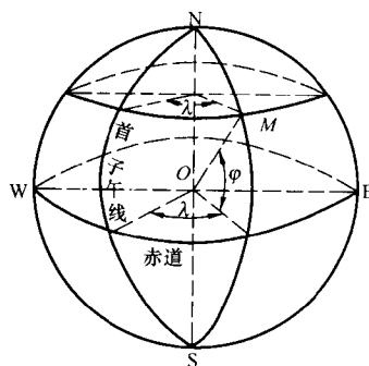
图 1-3 地理坐标
