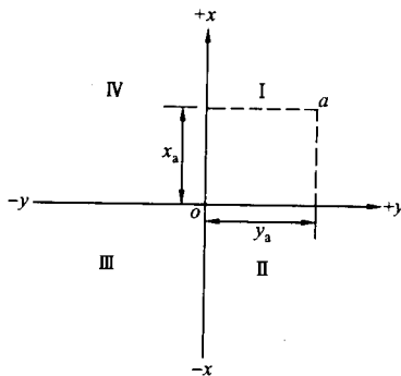
图 1-9 平面直角坐标
