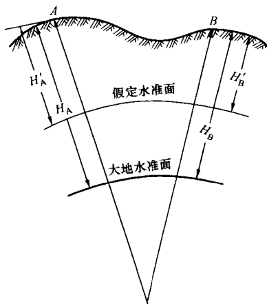
图 1-10 高程示意图
