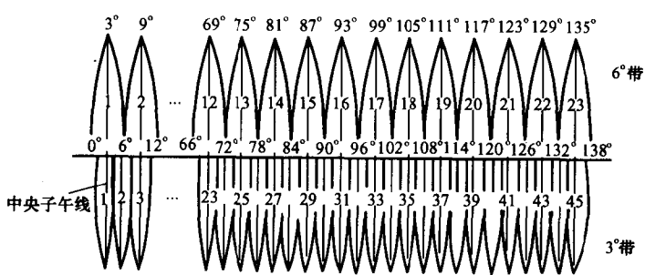
图 1-6 6^\circ 、 3^\circ 带投影
