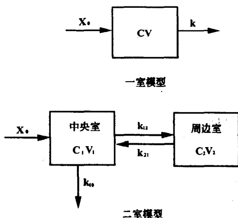
图 2.1 房室模型示意图
