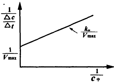
图 2.3 Lineweaver - Burk 法作图
