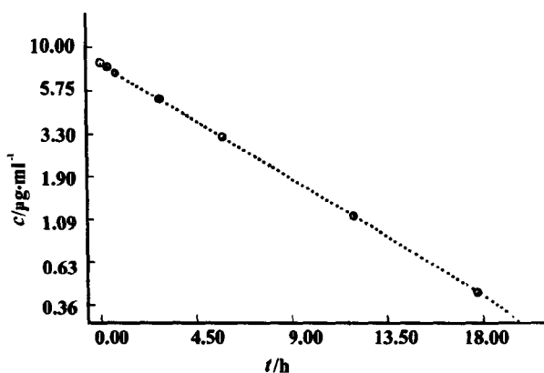
图 2.2 血药浓度 - 时间数据半对数作图(iv)
