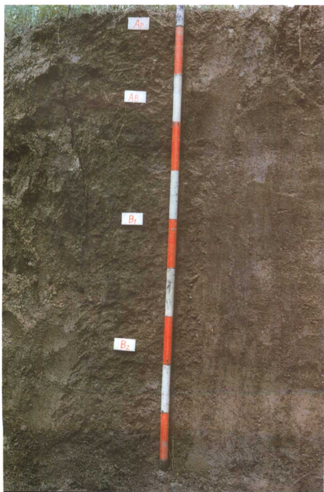
草甸暗棕壤剖面
