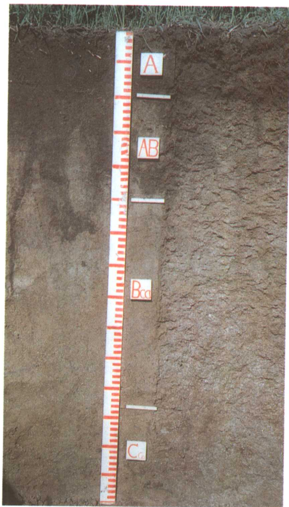
30 草甸黑钙土剖面
