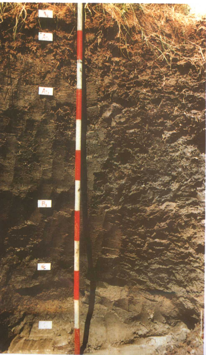
35 泥炭沼泽土剖面
