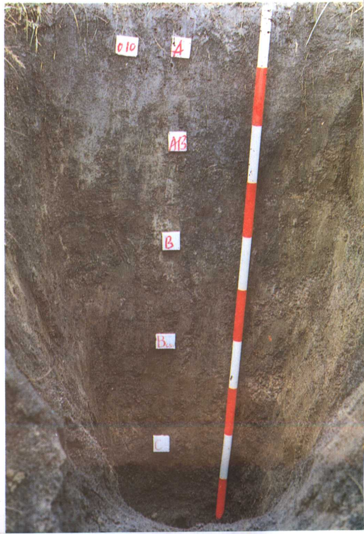
32 石灰性草甸土剖面
