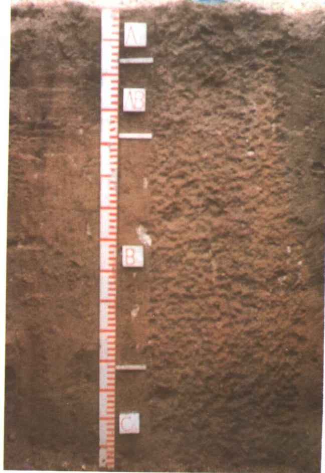
28 石灰性黑钙土剖面
