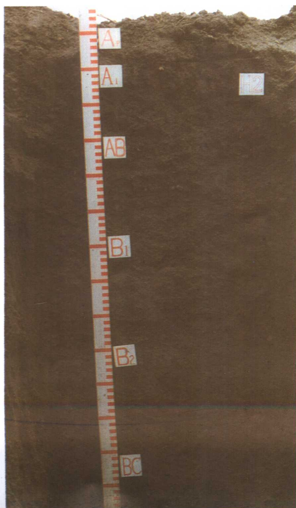
26 草甸黑土剖面
