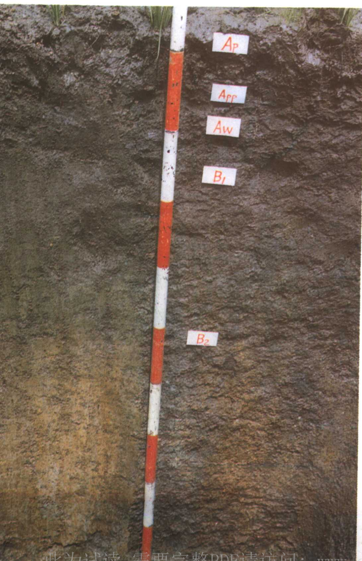
40 白浆土型淹育水稻土剖面
