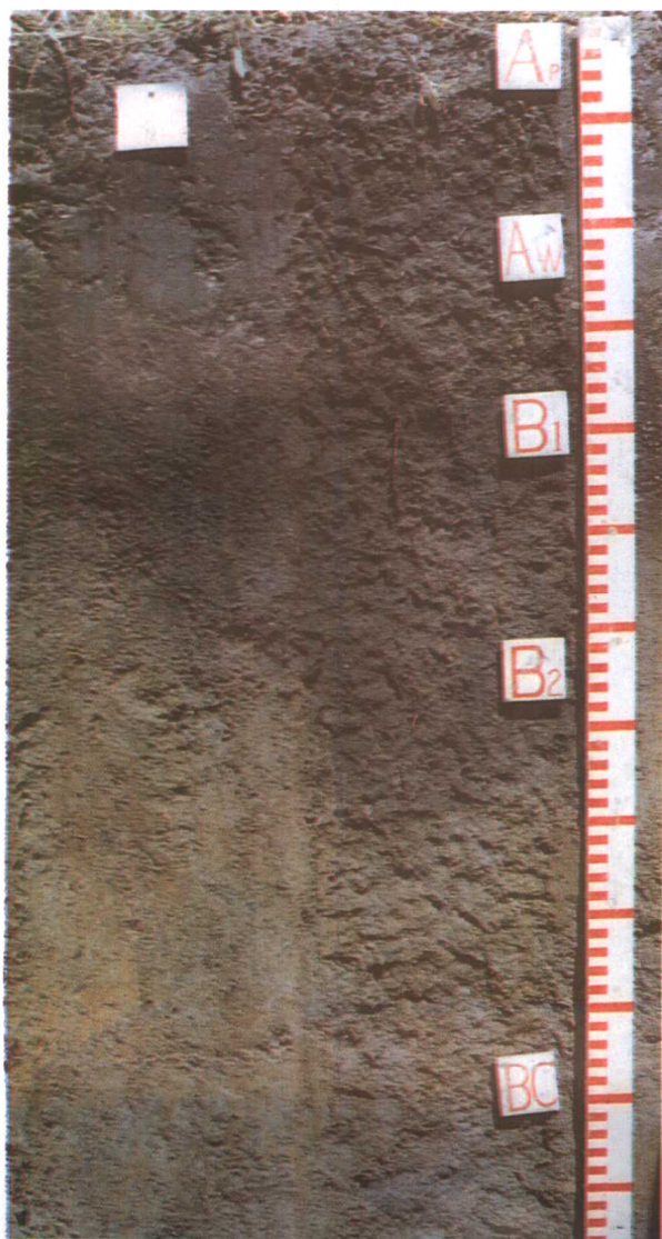
潜育白浆土剖面
