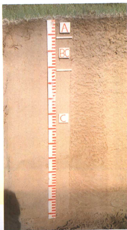
39 草甸风沙土剖面
