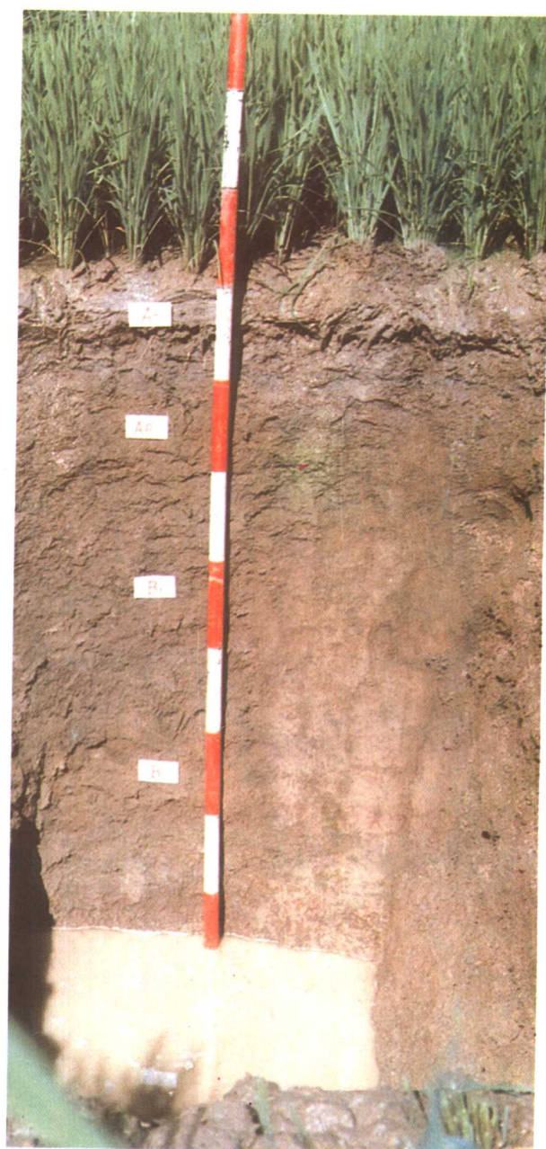
41 暗棕壤型淹育水稻土剖面
