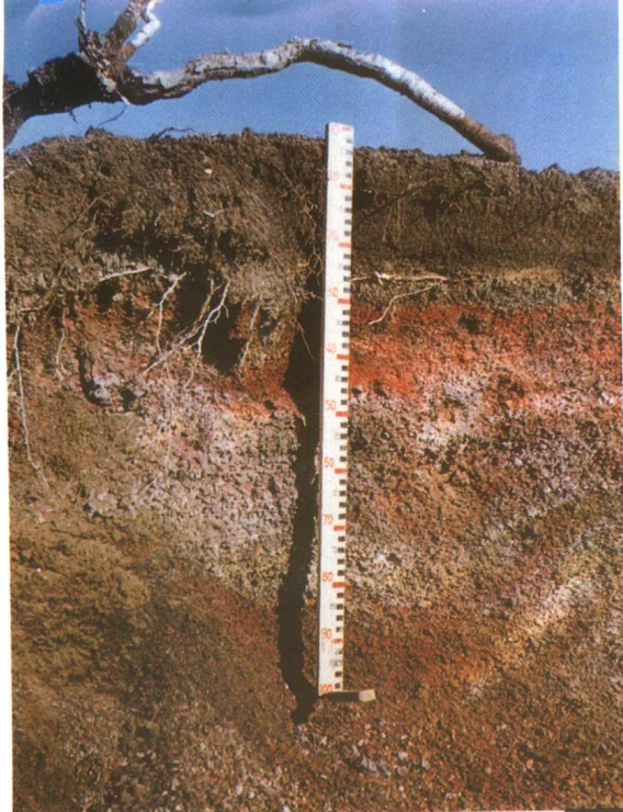
37 火山灰土剖面
