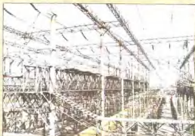
上海第一座户外高层结构 220 千伏变电站——万荣变电站
