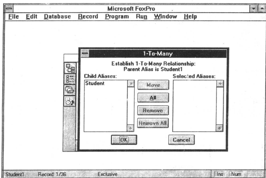
图 1 1—To—Many 对话
