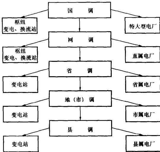
图1-2 电网分层控制示意图
